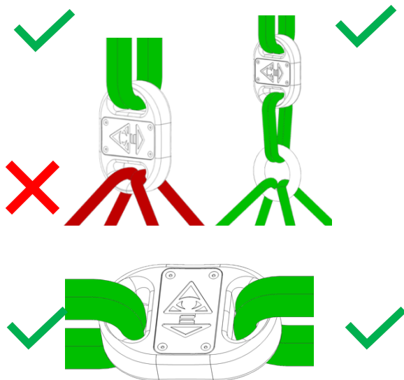
Abbildung 1 Falsches und richtiges Einschlaufen des Tauwerks
